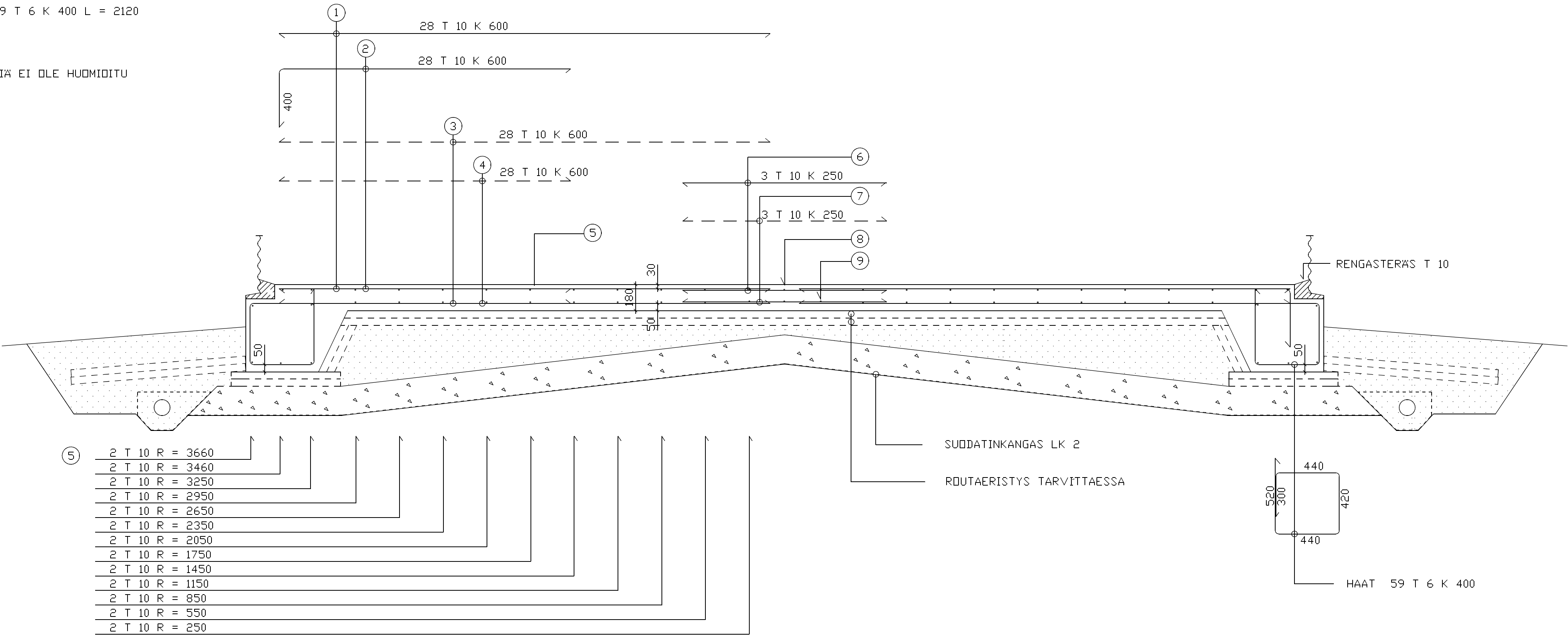
RAUDOITUS 1 / 20
