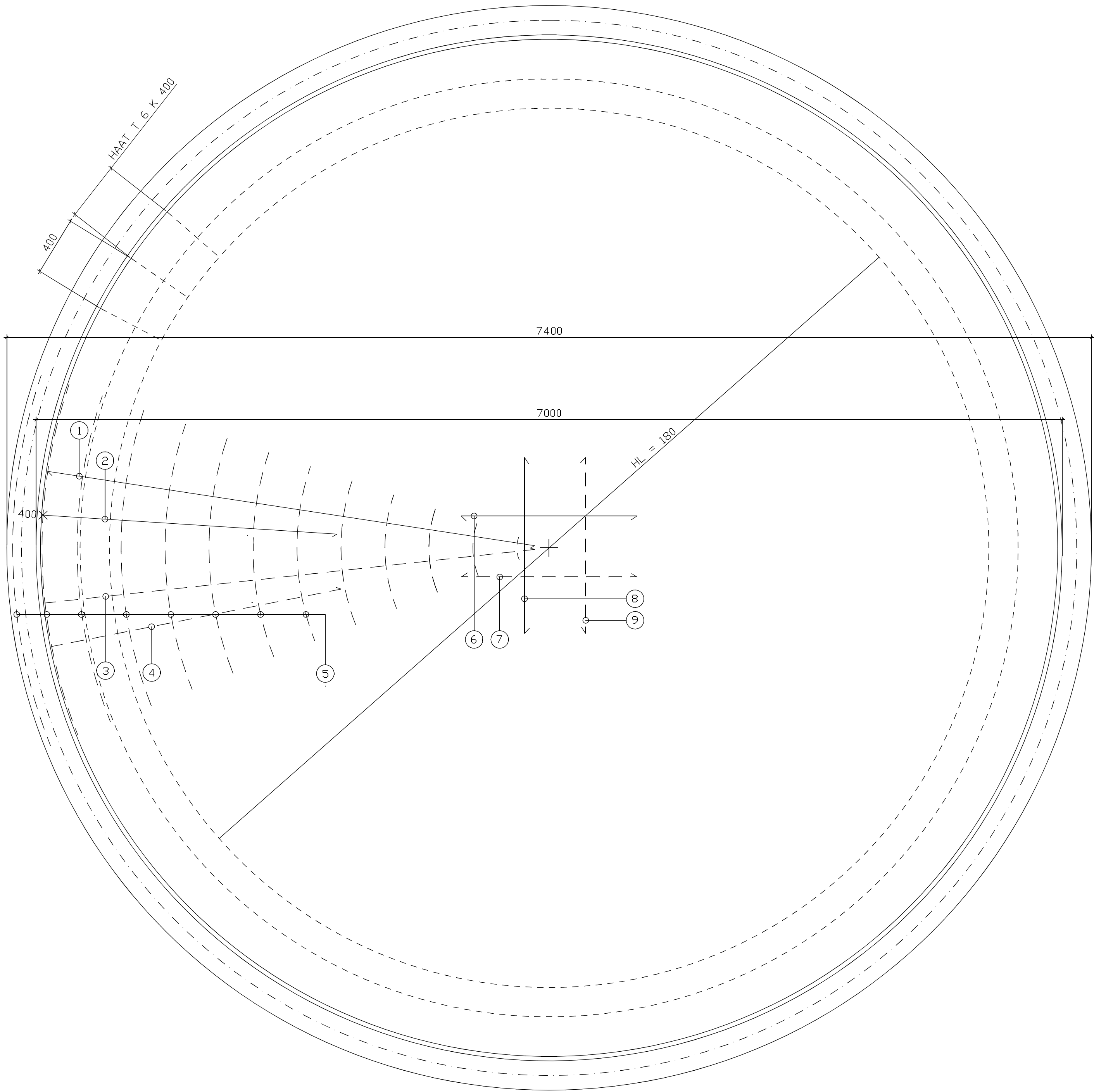
POHJA 1 / 20
