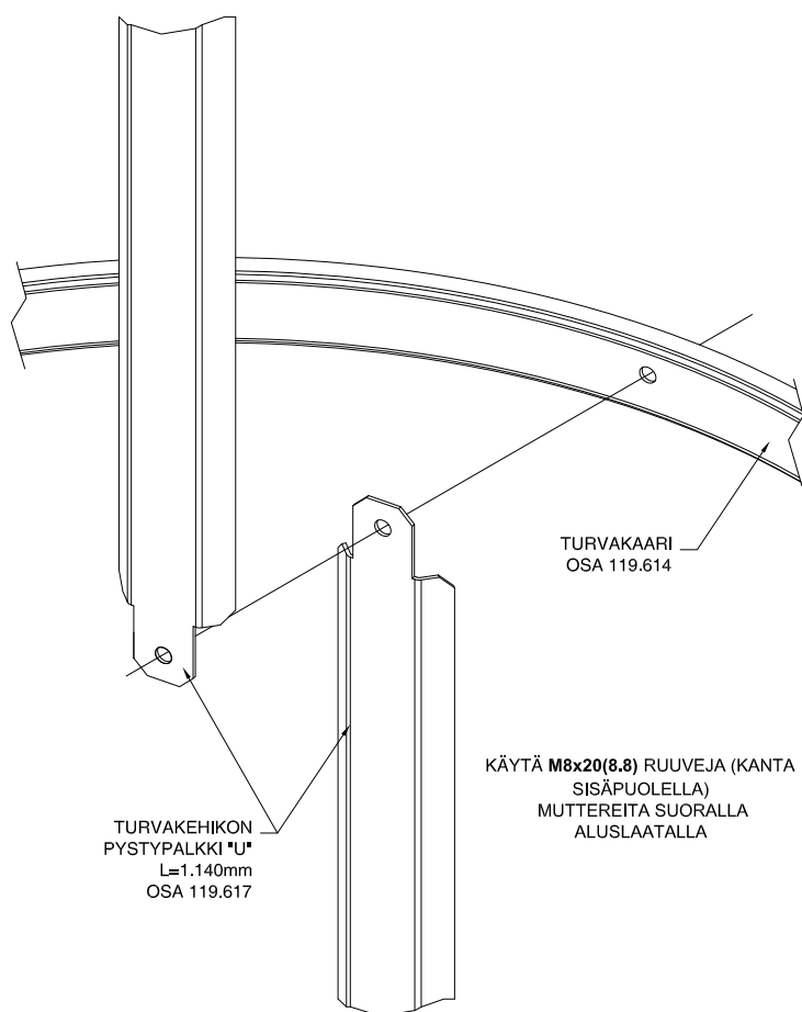
DETALJI 3
