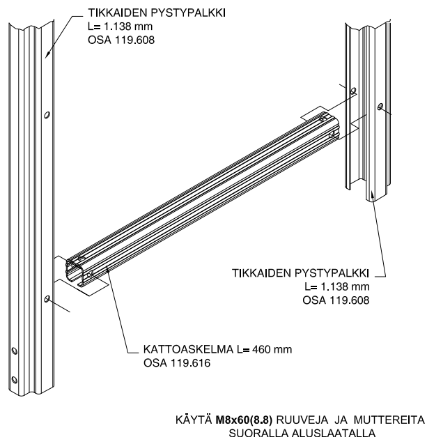
DETALJI 4
