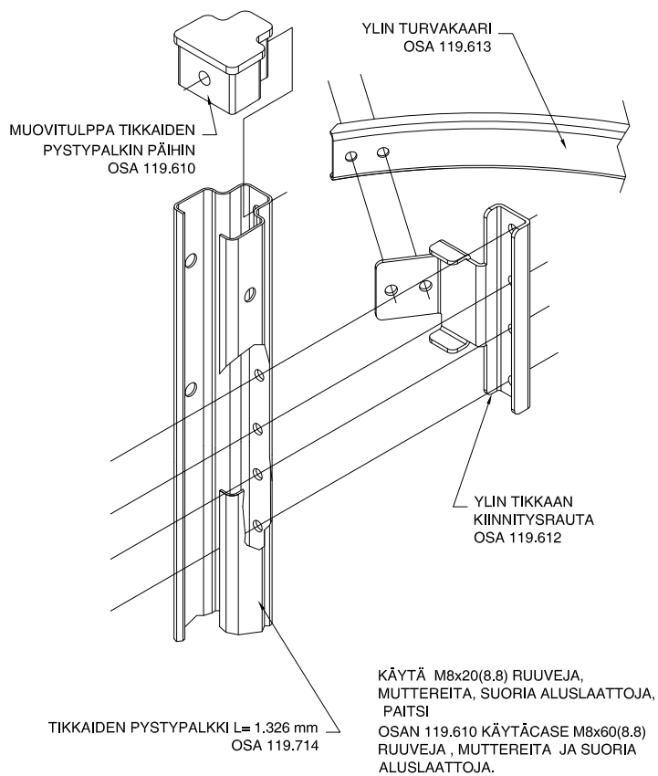
DETALJI 1
