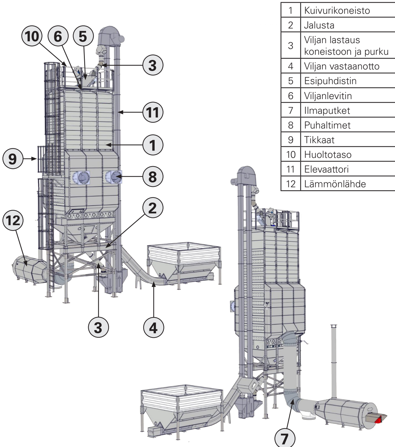
Kuva 3.1. Viljankuivaamon tärkeimmät osat
