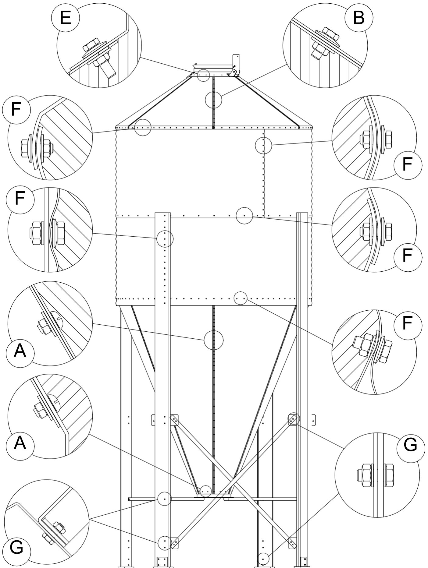
Liitostyypit ja niiden eri asennot. Pulttien, muttereiden ja aluslevyjen tekniset tiedot.
