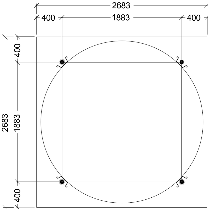
ANKKURIPULTTIEN JAKAUTUMINEN PERUSTUKSEEN
