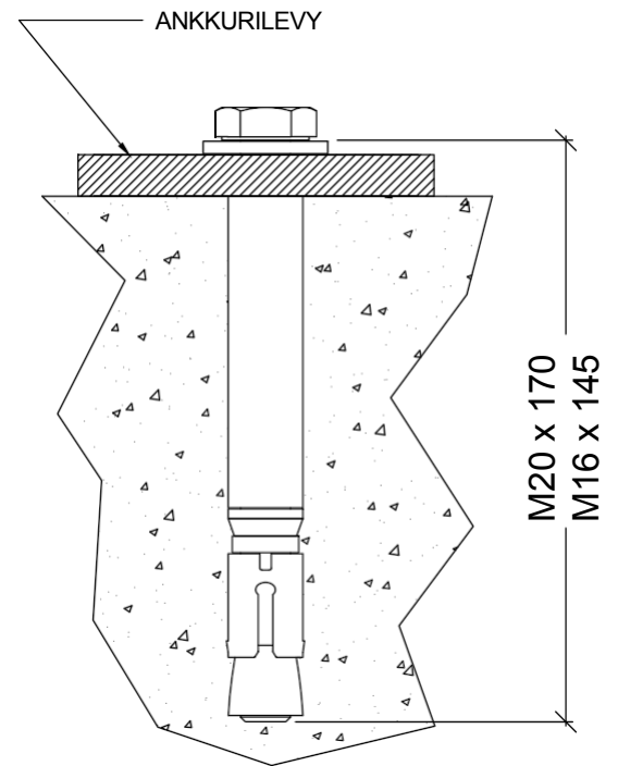
KIILA-ANKKURI BETONIIN KIINNITTÄMISTÄ VARTEN
