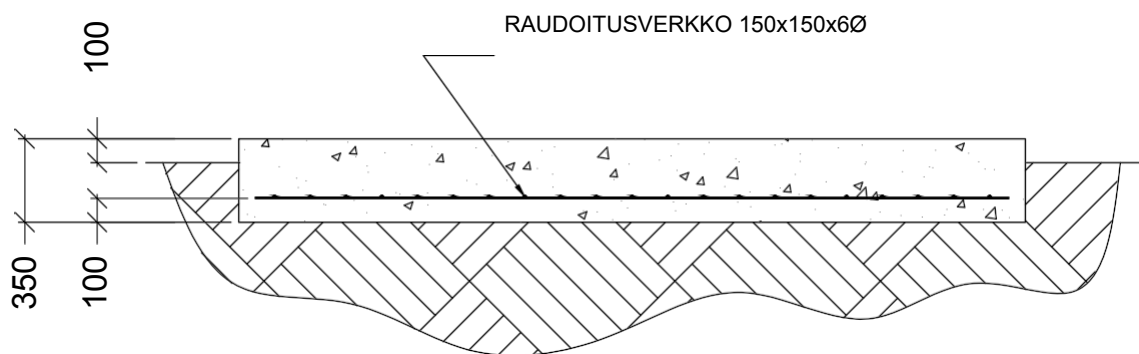
PERUSTUKSEN POIKKILEIKKAUS
